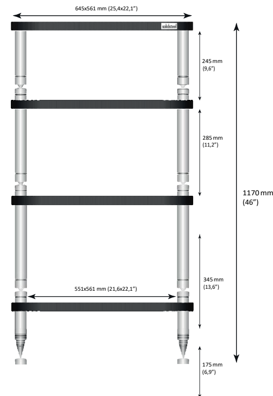
HF-4 Colossus [345/285/245] - Special Hyperspike AV Rack
