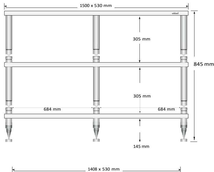
HFW-3XL [305/305] - Special Hyperspike AV Rack
